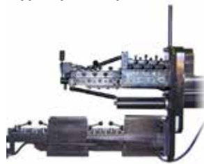
3-positions flipper for straightener Flipper 3 posizioni per raddrizzafilo
