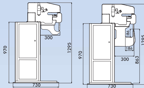
Accessorio n° 2 - Accessory n° 2 (mm)
