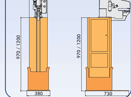
Basamento sollevabile (mm) Risable Stand
