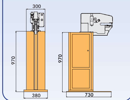
Basamento fisso (mm) Fixed Stand
